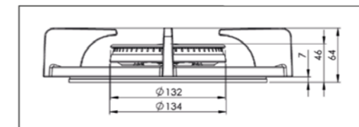
WOK-/SIMMER BURNER
